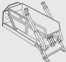
MOLOZ KONTEYNER YÜKLEYİCİ SKIP LOADER
